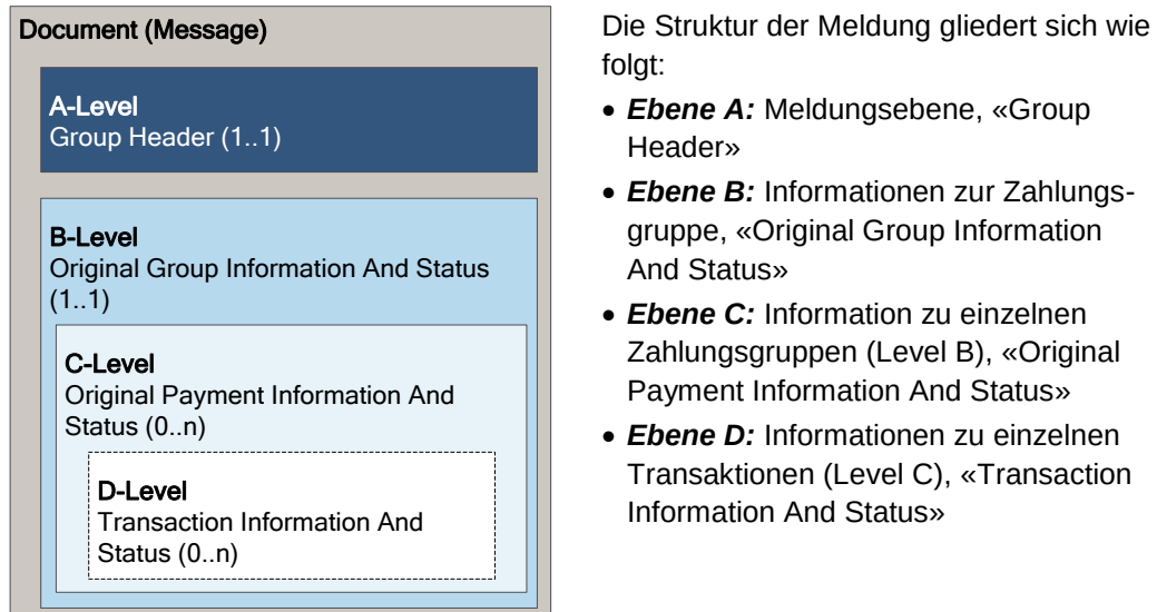
Abbildung 4: Meldungsstruktur Payment Status Report
