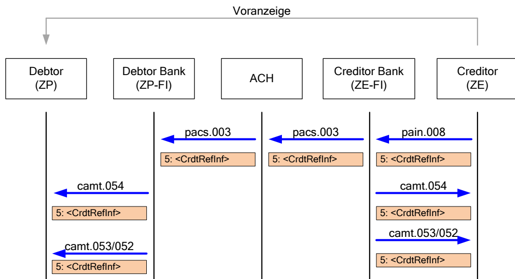
Abbildung 14: Strukturierte Referenz im Direct Debit (pain.008)
