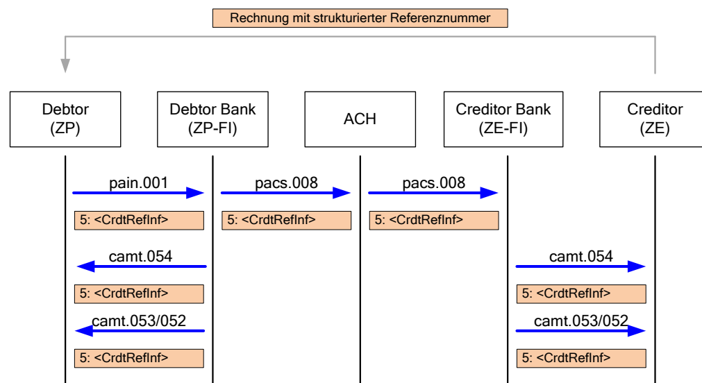
Abbildung 13: Strukturierte Referenz im Credit Transfer (pain.001)
