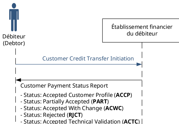
Illustration 4: Synthèse du statut possible dans le Status Report
