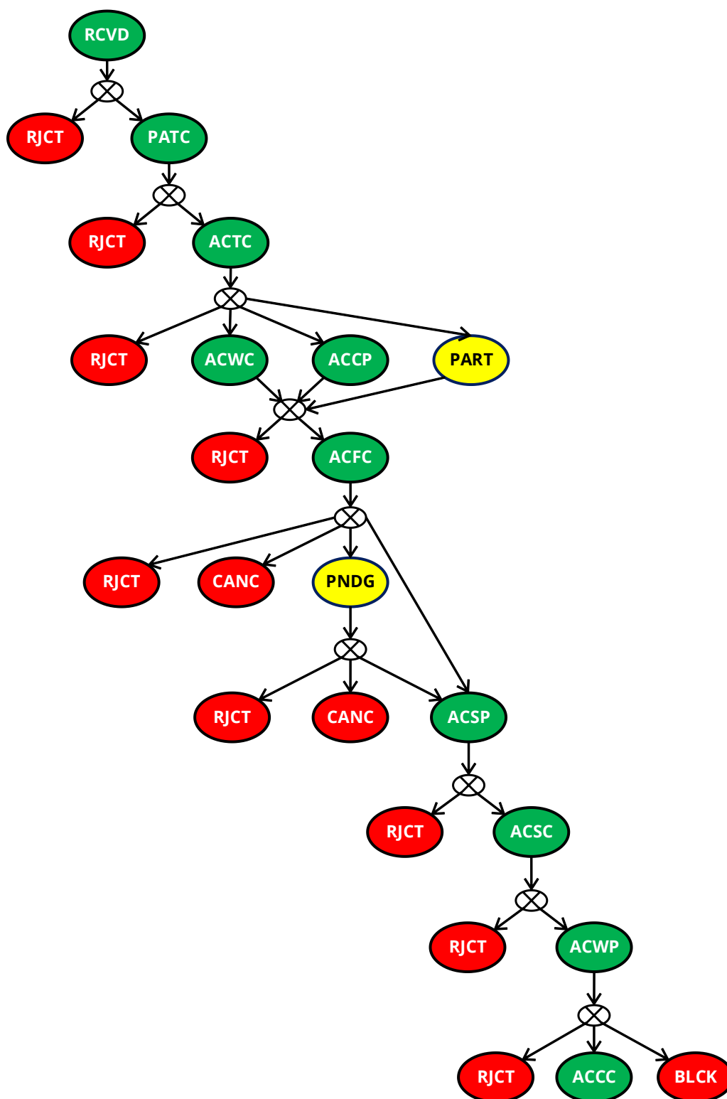
Illustration 13: Séquences de statuts de pain.002
