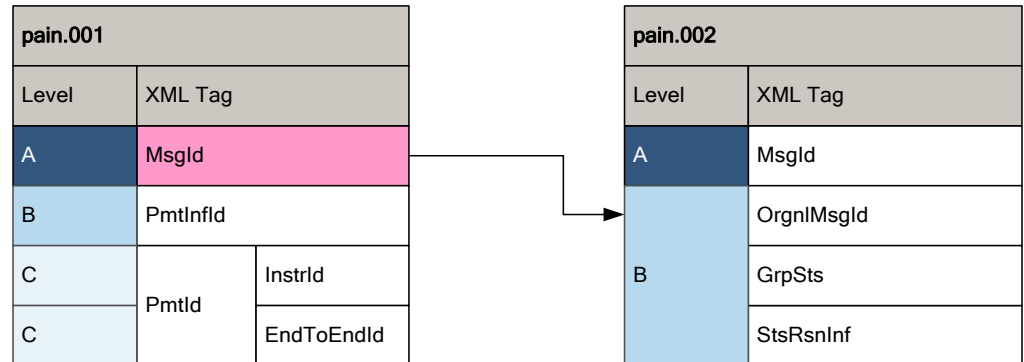
Illustration 6: Erreur au «pain.001» A-Level – Références dans «pain.002»
