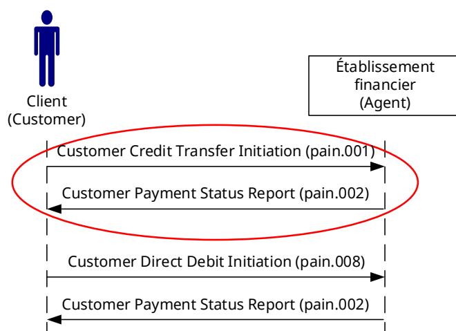
Illustration 1: Synthèse des flux de messages Payment Initiation
