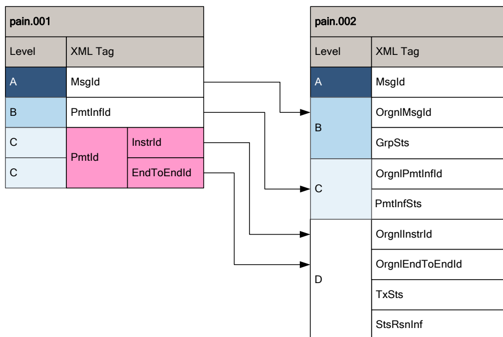
Illustration 8: Erreur au «pain.001» C-Level – Références dans «pain.002»
