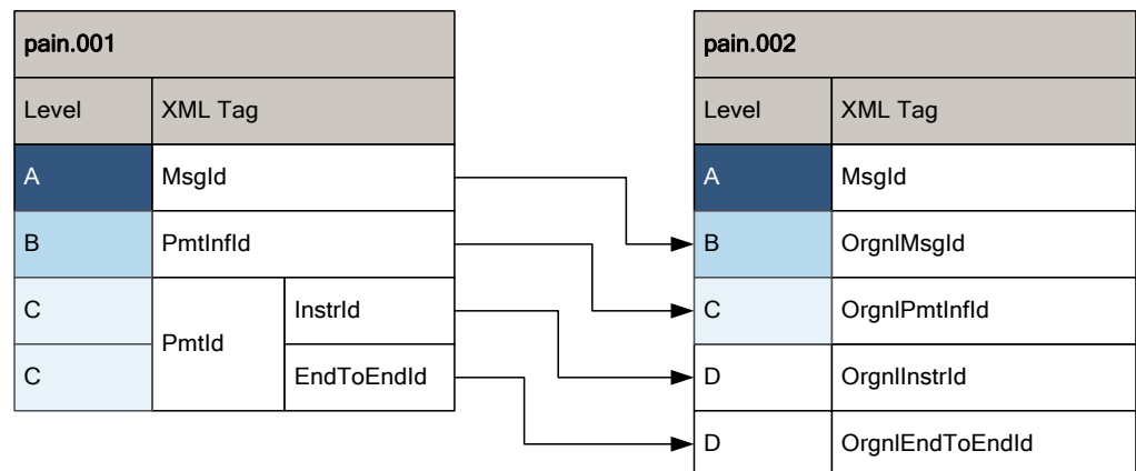
Illustration 5: Schéma de base pour le mapping «pain.001» vers «pain.002»
