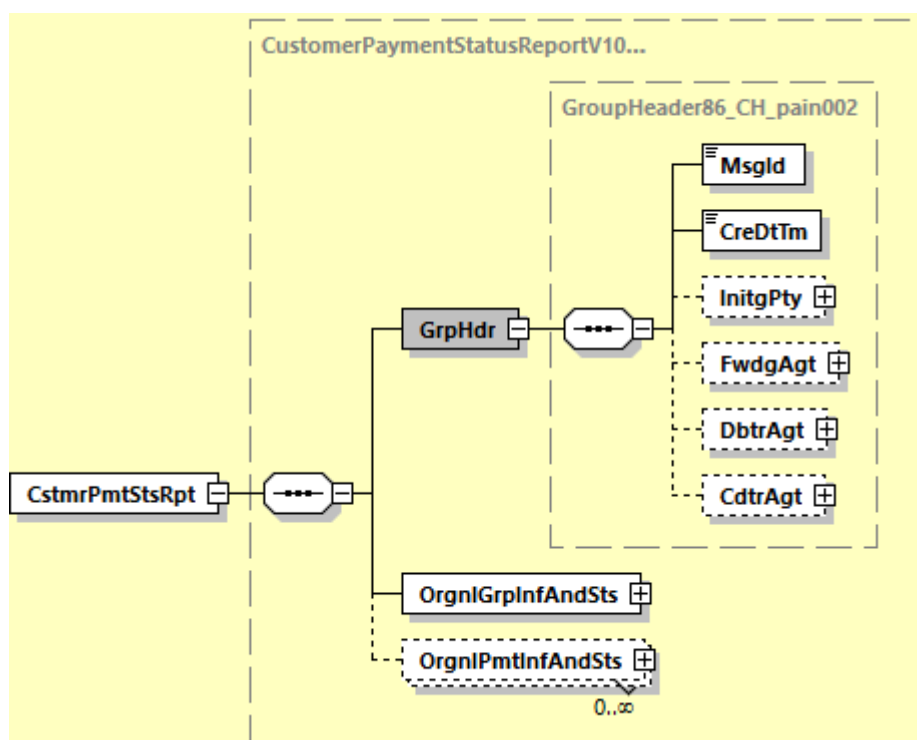
Illustration 2: Exemple d'un affichage de message XML sous forme graphique
