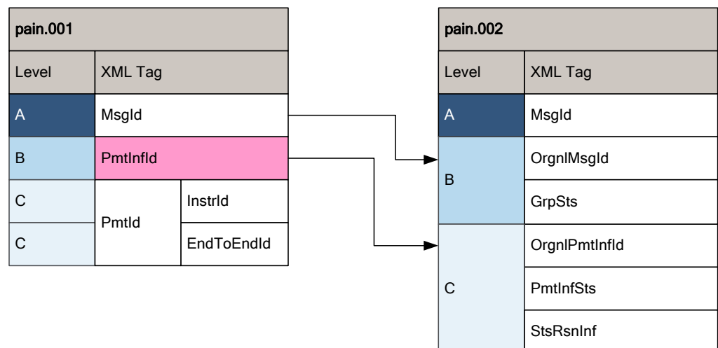
Illustration 7: Erreur au «pain.001» B-Level – Références dans «pain.002»
