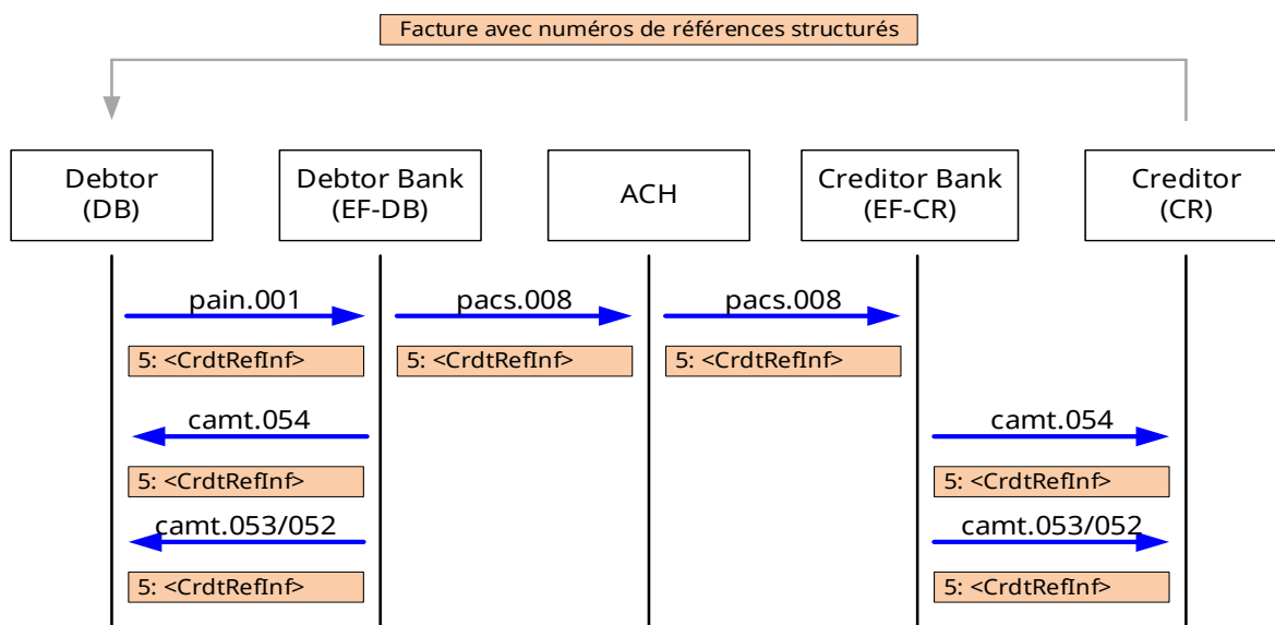
Illustration 10: Référence structurée dans le Credit Transfer (pain.001)
