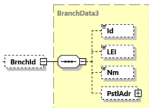
Illustration 6: Éléments de données complémentaires pour l'identification de succursales des établissements financiers (générique)
