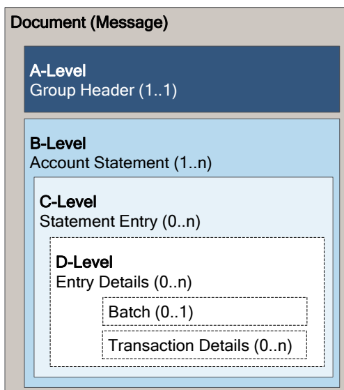
Abbildung 12: Meldungsstruktur von Cash-Management-Meldungen (camt.053)
