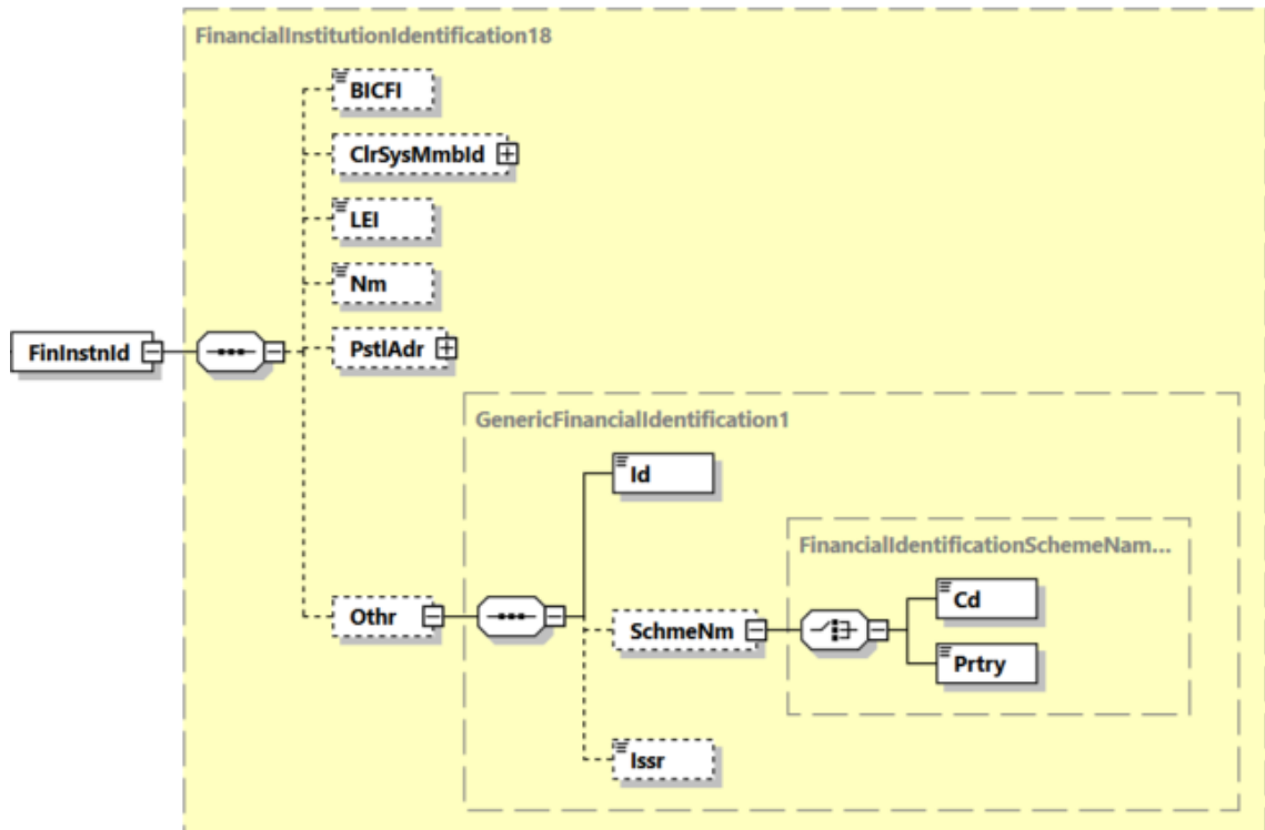
Abbildung 5: Datenelemente zur Identifikation von Finanzinstituten (generisch)
