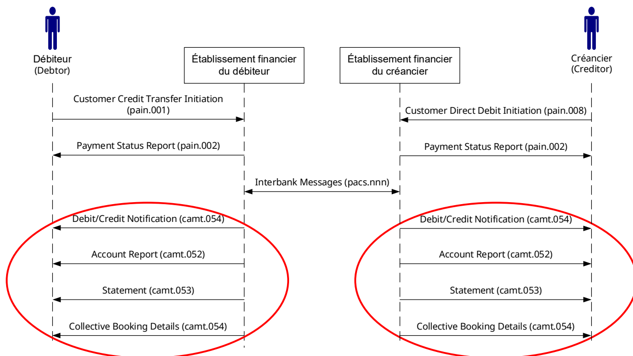
Illustration 1: Ordres de paiement et Cash Management (reporting) avec ISO 20022
