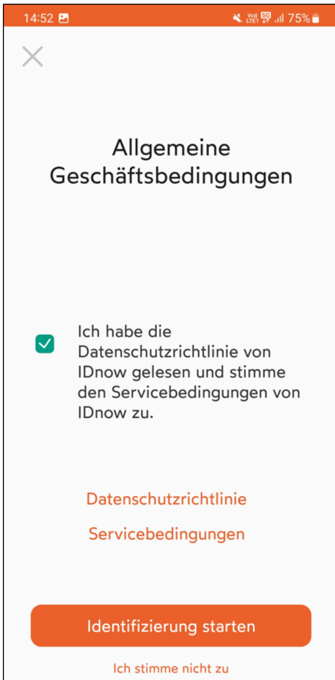
Figura 6, condizioni generali
